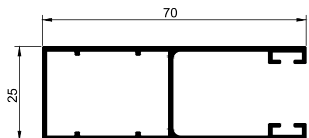
ES.35 Calha Lateral
