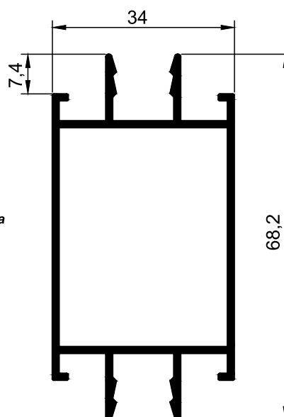
DI.03 Montante/Travessa
