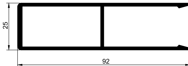
ST.33 Régua Superior Taipal
