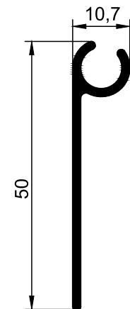
ES.06 Terminal Lâmina
