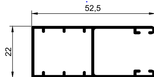
ES.34 Calha Lateral
