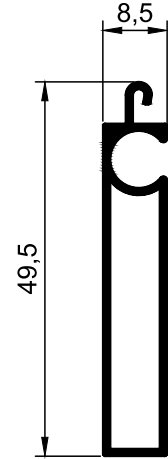
ES.02 Lâmina
