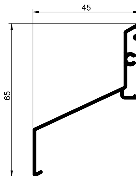
LS.11 Lâmina 45*65mm
