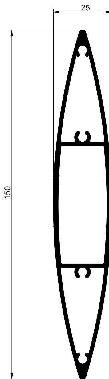
ST.78 Lâmina Triângular
