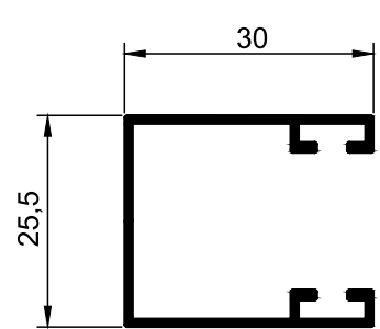
ES.31 Calha Lateral
