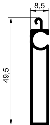
ES.05 Lâmina
