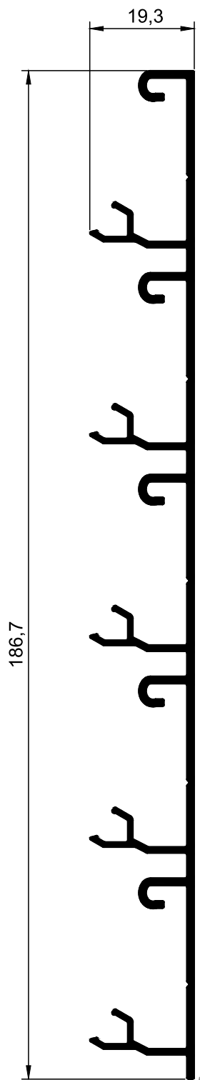
LS.23 Fixador Lâmina
