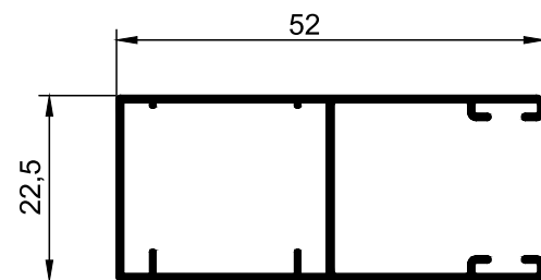
ES.33 Calha Lateral
