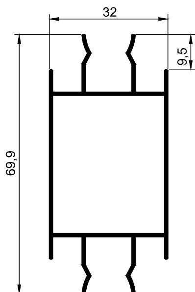
DI.03 Montante/Travessa
