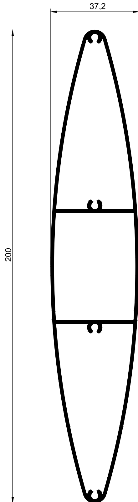
LS.03 Lâmina Solar 200mm
