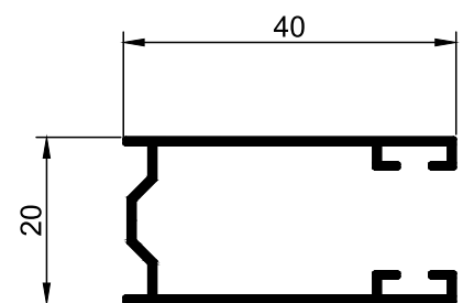
ES.07 Calha Lateral
