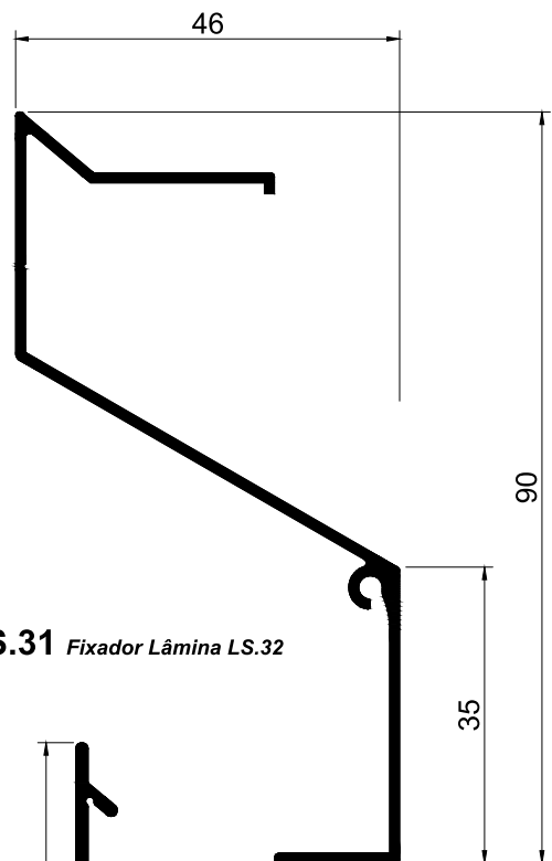
LS.32 Lâmina 46*90mm
