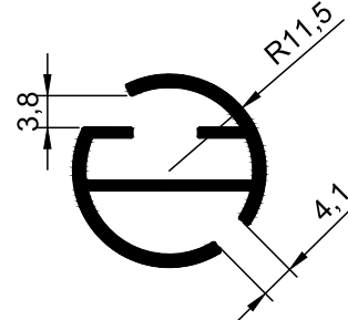
ES.62 Base Redonda
