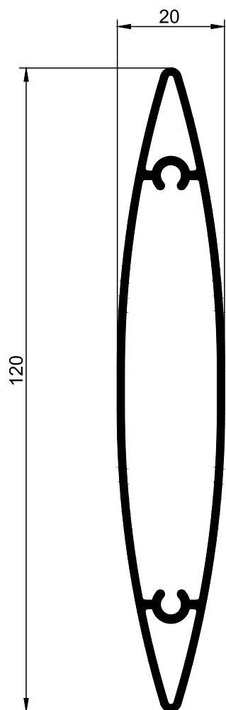
LS.01 Lâmina Solar 120mm
