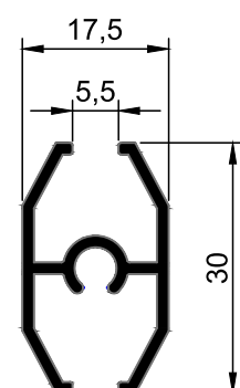
V.07 Vidrinhos
