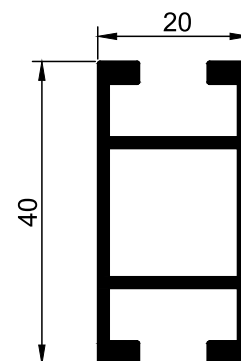
BC.04 Perfil Mobiliário Travessa Dupla
