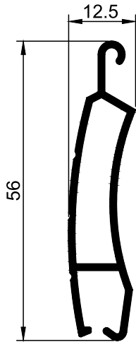
ES.01 Lâmina
