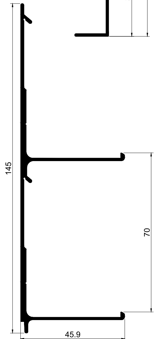
LS.31 Fixador Lâmina LS.32
