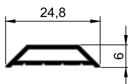
V.08 Vidrinhos
