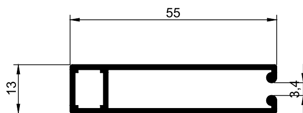
ES.56 Calha Lateral
