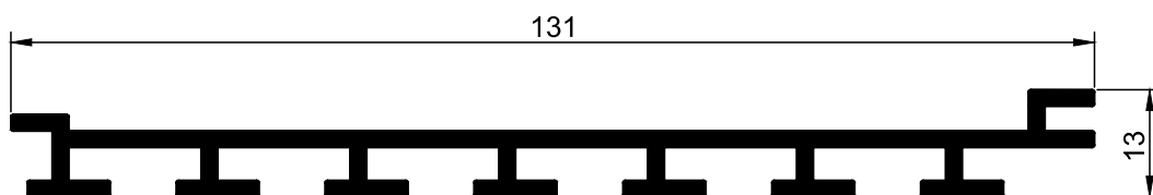
ST.14 Prateleira
