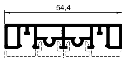
RM.12 Rede Mosquiteira Travessa
