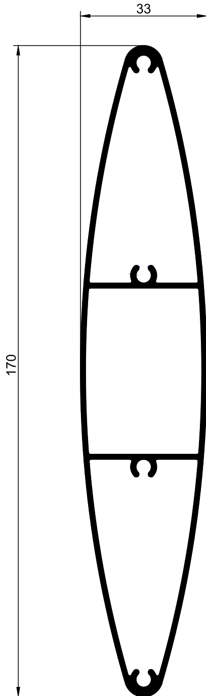
LS.02 Lâmina Solar 170mm
