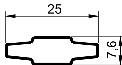
V.01 Vidrinhos
