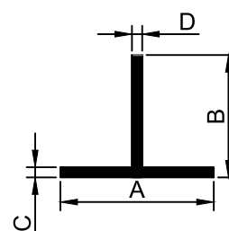
Perfil em T
