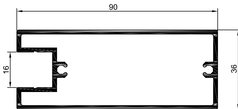
PT.106 Travessa Superior/Inferior
