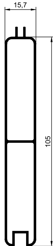
W.29 Lâmina
