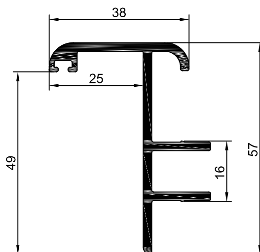
PT.108 Inversor
