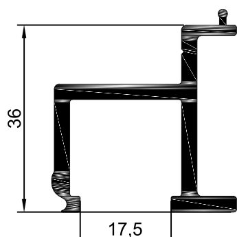
PT.112 Callha Lateral
