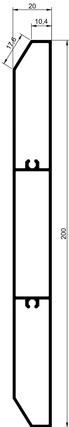
W.42 Lâmina
