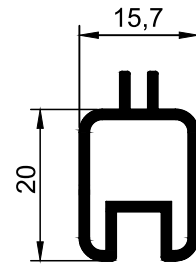
W.37 Lâmina
