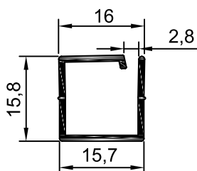
PT.109 Redutor
