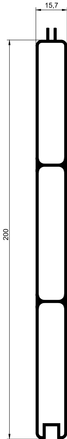
W.30 Lâmina
