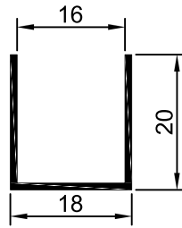
U.29 Calha "U"
