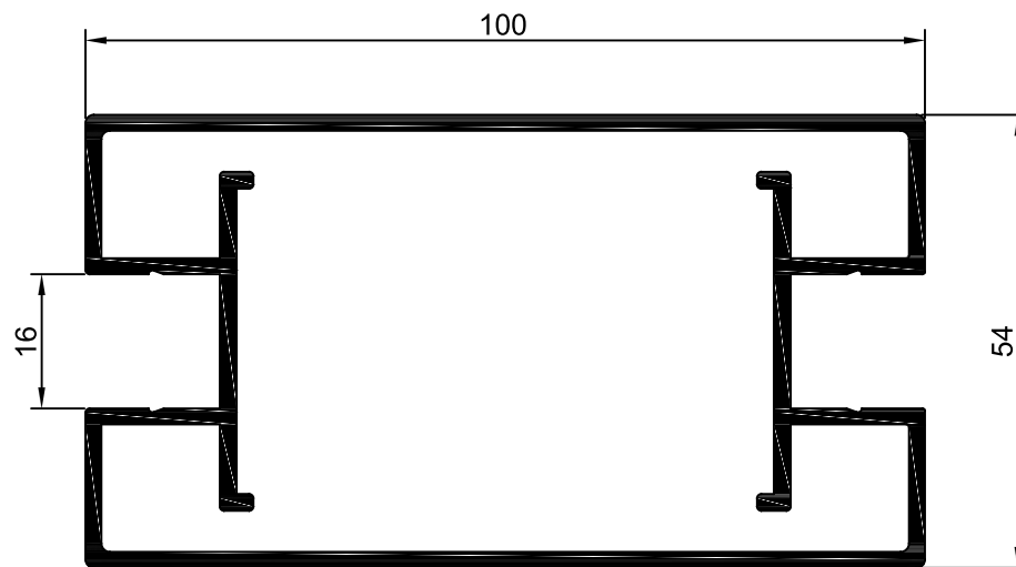
PT.105 Prumo Vertical
