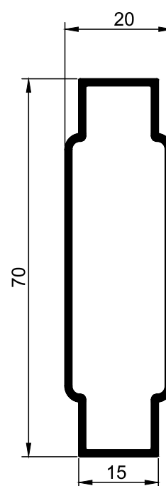
W.42 Lâmina
