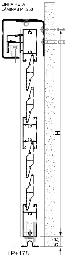
LINHA RETA LÂMINAS W.36
