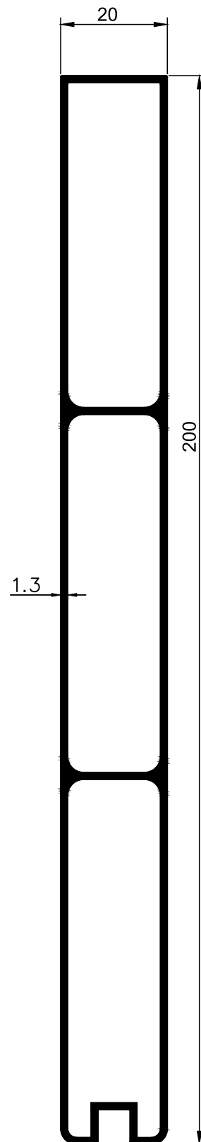
W.46 Lâmina
