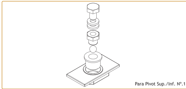
Para Pivot Sup./Inf. Nº.1
