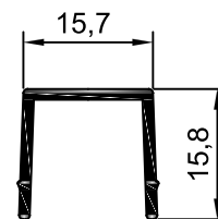
PT.109A Tapa Junta
