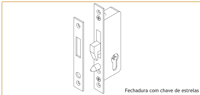
Fechadura com chave de estrelas
