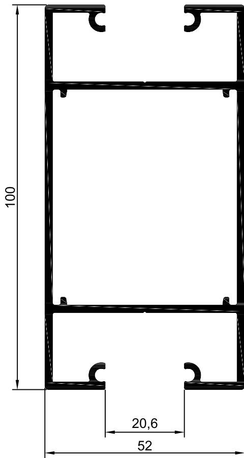
PT.241 Prumo Vertical
