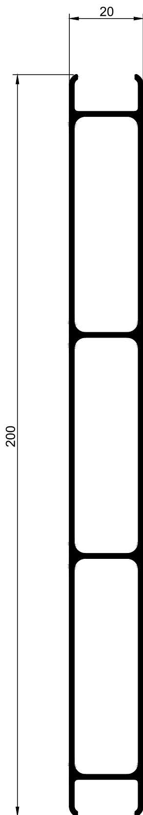
W.39 Lâmina
