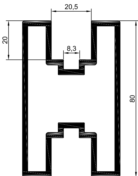
PT.103 Travessa
