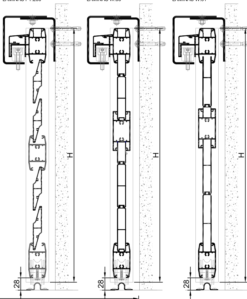
LINHA REDONDA LÂMINAS PT.250
