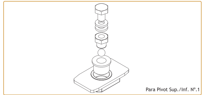
Para Pivot Sup./Inf. Nº.1
