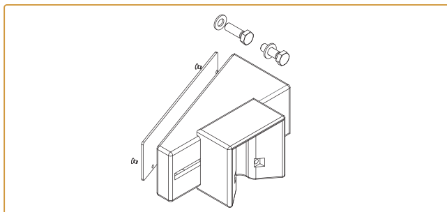
FECHO LATERAL REG. 21060
